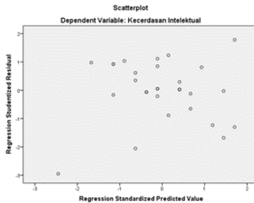
Gambar 2. heteroskedastisitas
